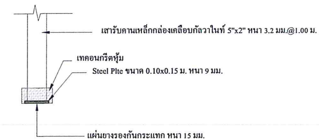
ขยาย 1 มาตราส่วน 1:25
