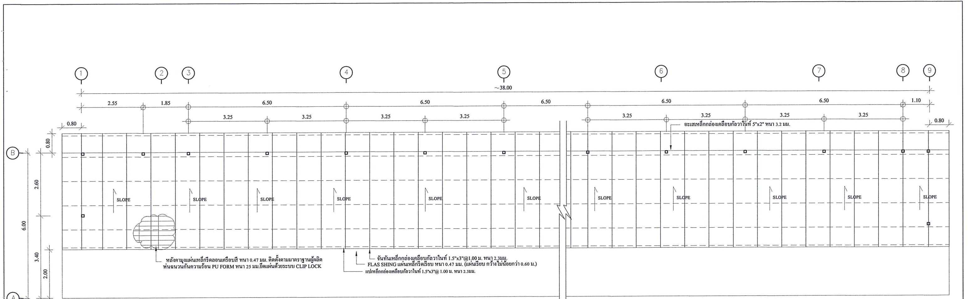
แบบ โครงหลังคา มาตราส่วน 1:100
