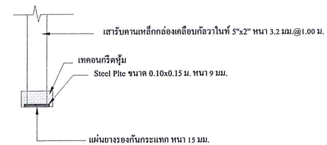
ขยาย 1 มาตราส่วน 1:25
