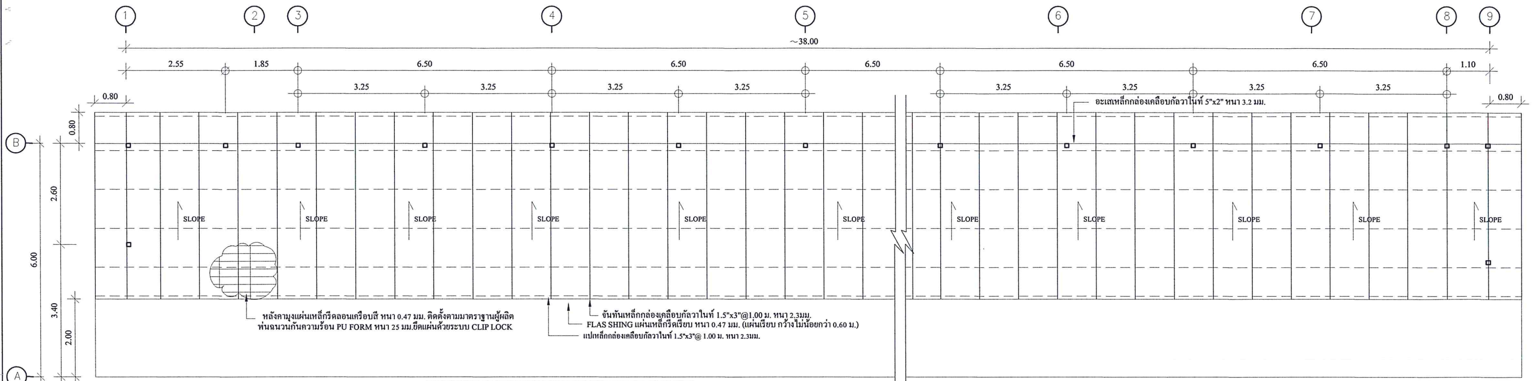
แบบ โครงหลังคา มาตรฐาน 1:100
